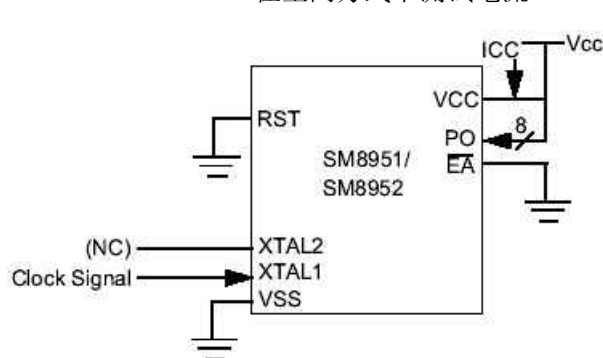
VCC 在空闲方式下测试电流
